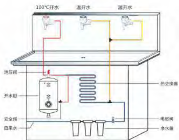
水流路径示意 图1 Water flow path diagram
